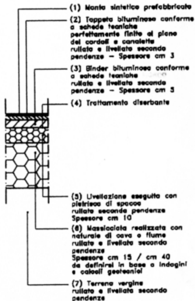
SEZIONE TIPO SOTTOFONDO
